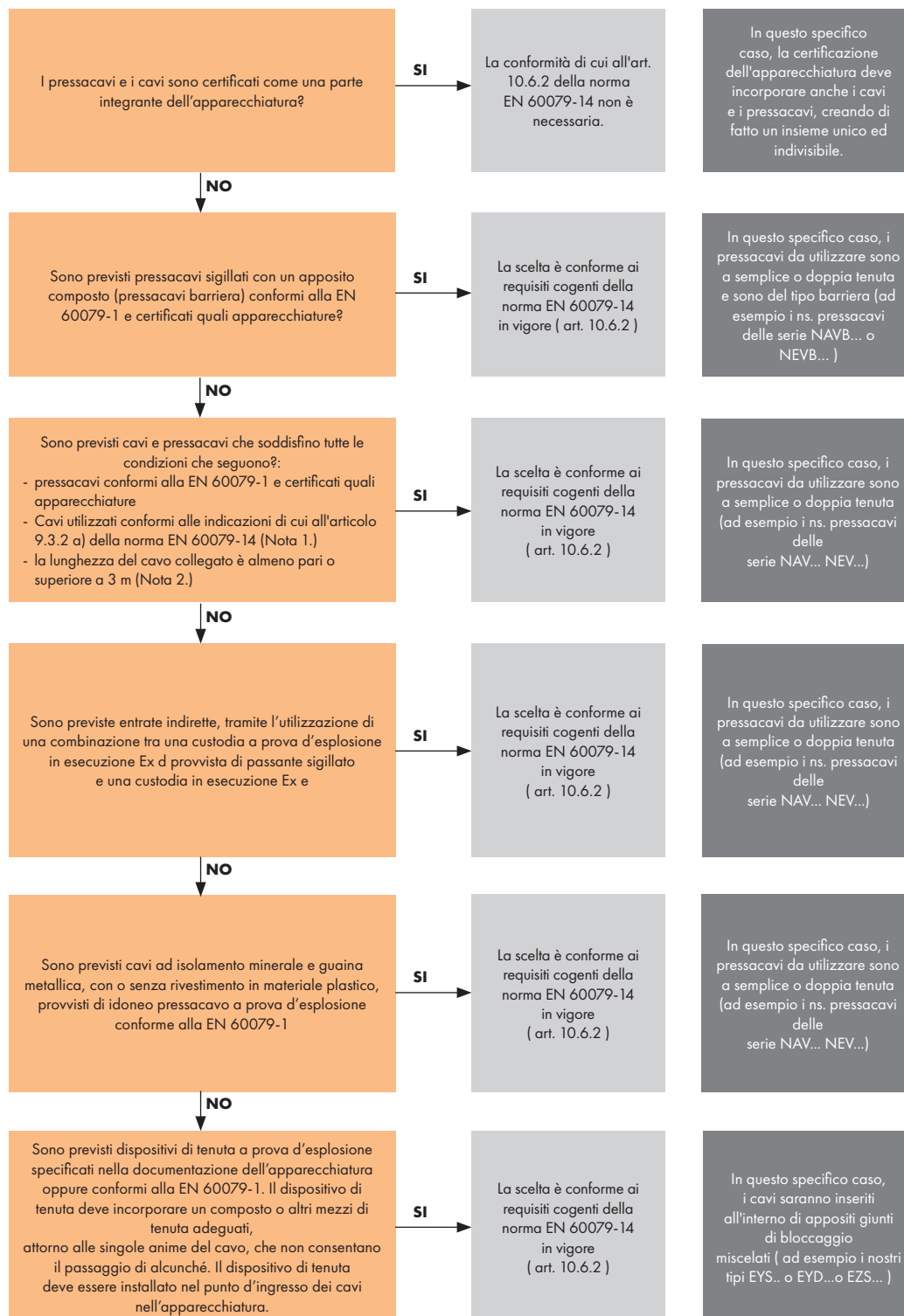
FIG.8 Diagramma di flusso per una corretta selezione dei sistemi di ingresso cavi in custodie a prova di esplosione in esecuzione Ex d.
