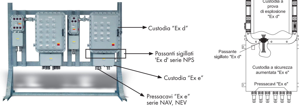
FIG.11 Esempio di impianto in cavo con entrata indiretta
