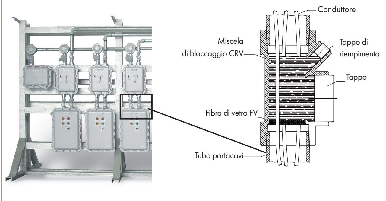
FIG.9 Esempio di impianto realizzato in tubo. Tra una custodia e l'altra si notano i giunti di bloccaggio serie EYS
